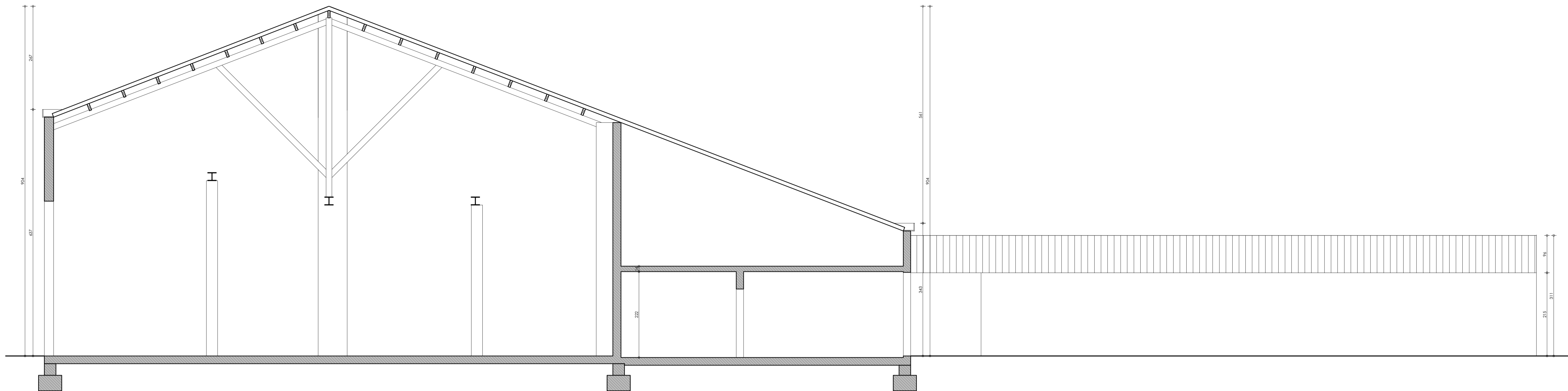
BT snede CD schaal 1:50
