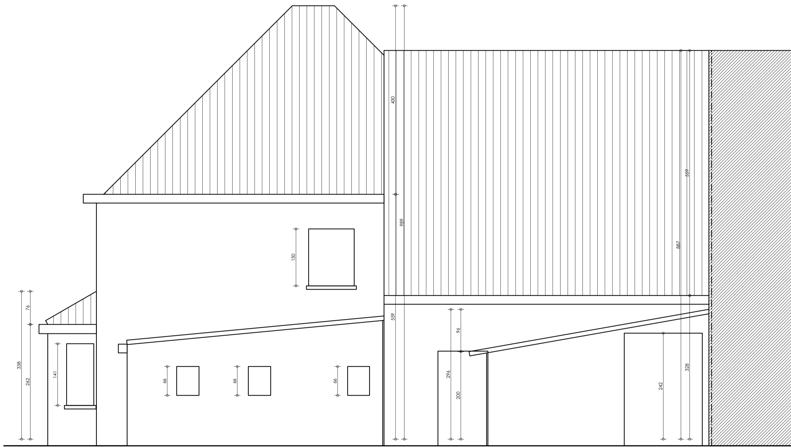
BT achtergevel schaal 1:50
