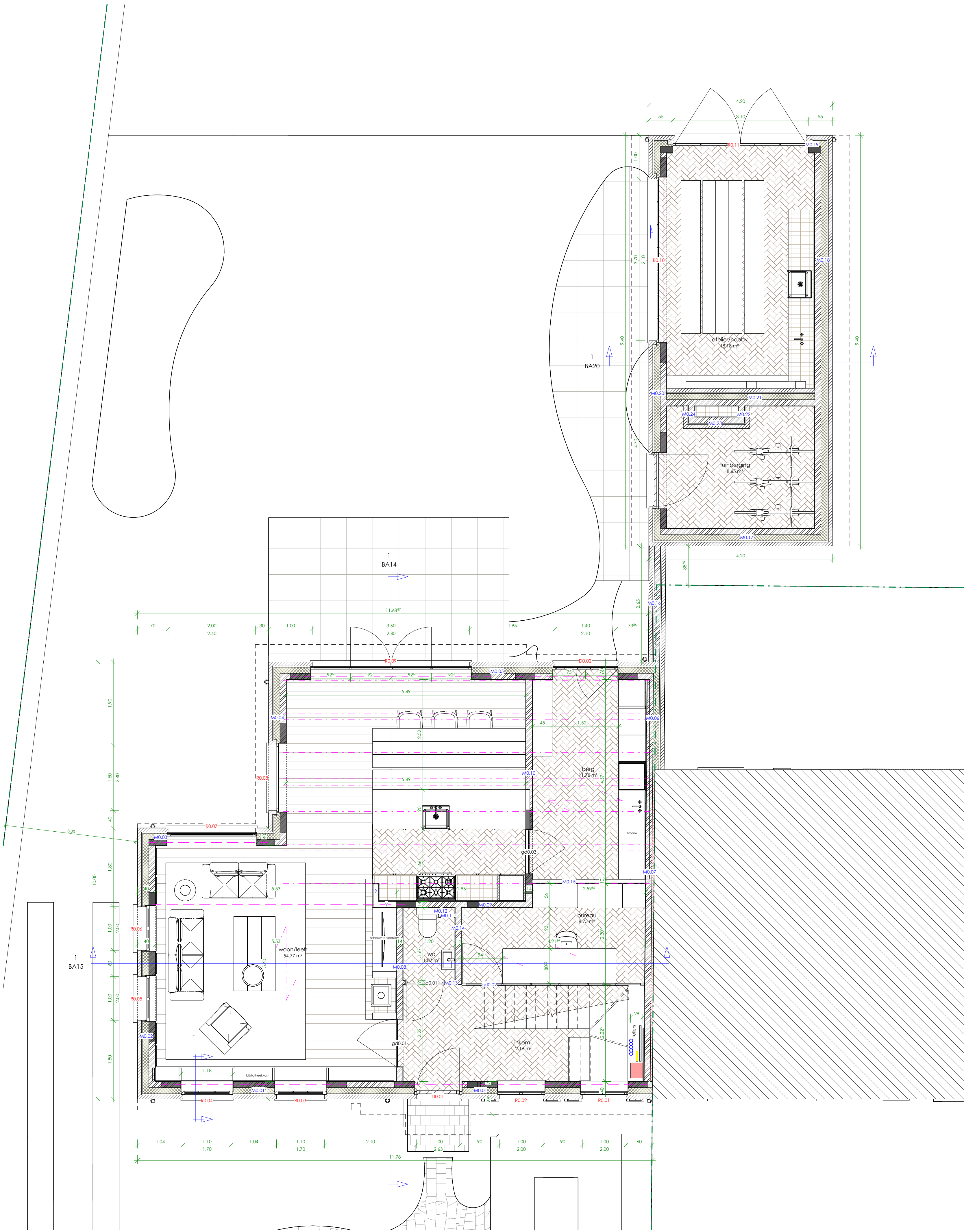
1 00_gelijkvloers - BA 1 : 50 0 5m
