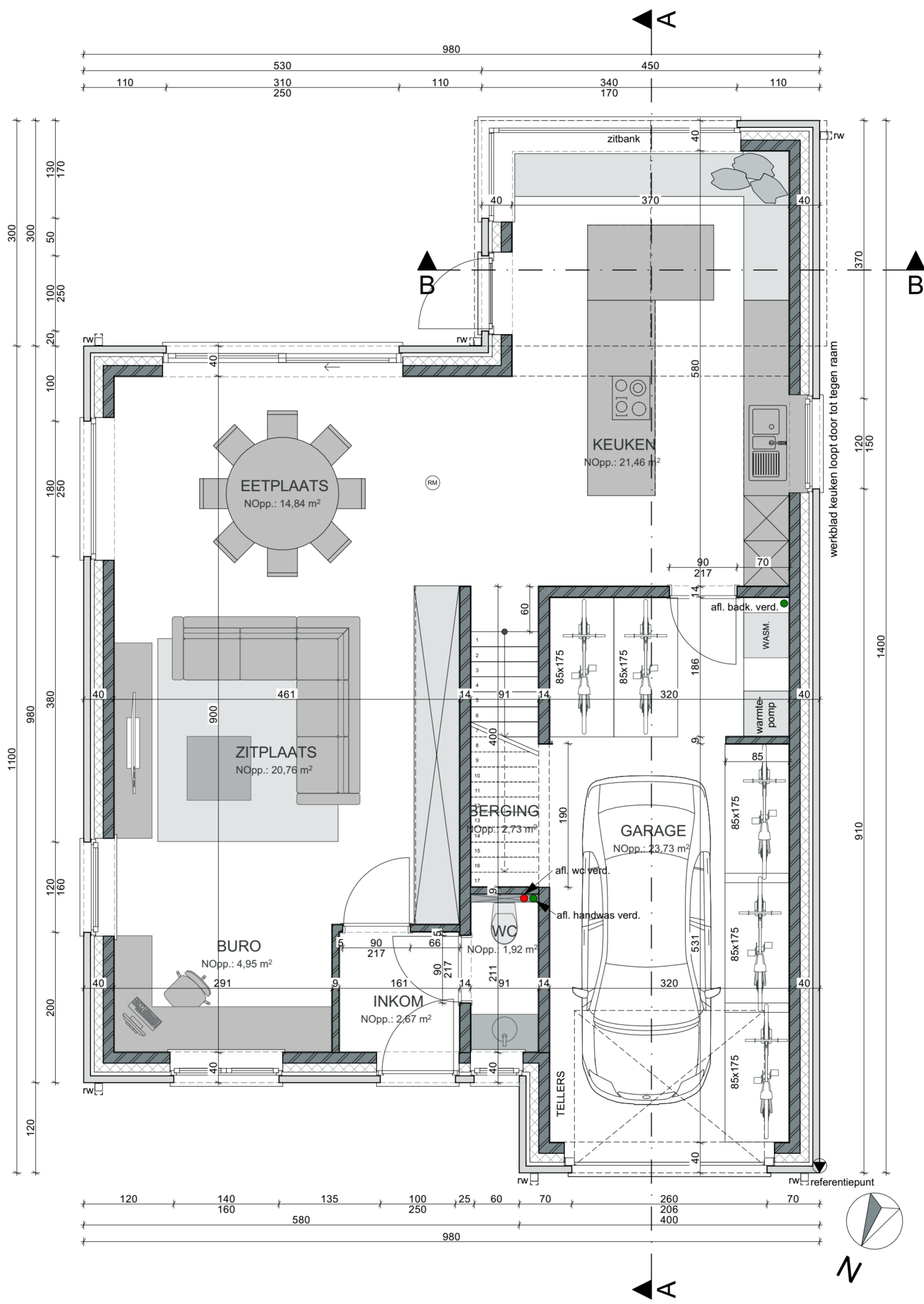
GRONDPLAN GELIJKVLOERS
