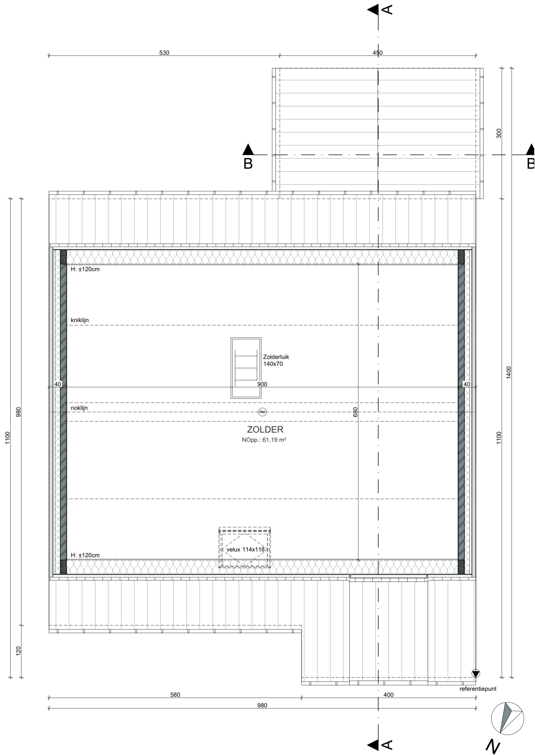
GRONDPLAN ZOLDERVERDIEP
