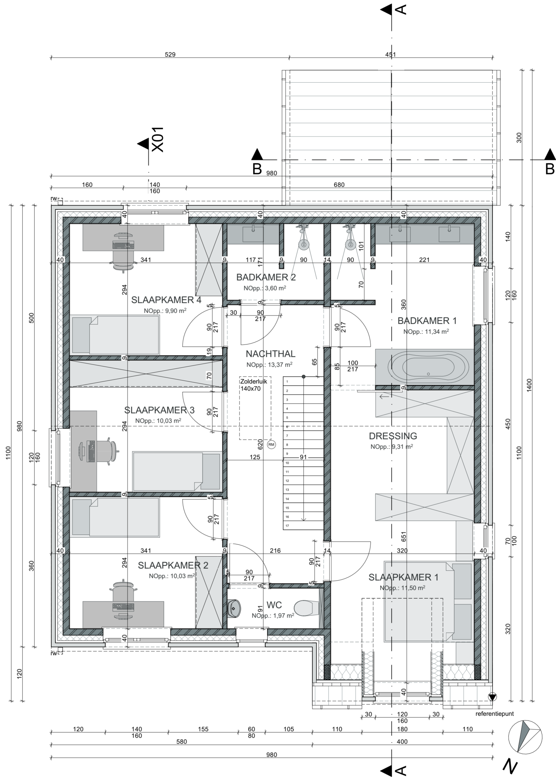
GRONDPLAN VERDIEPING
