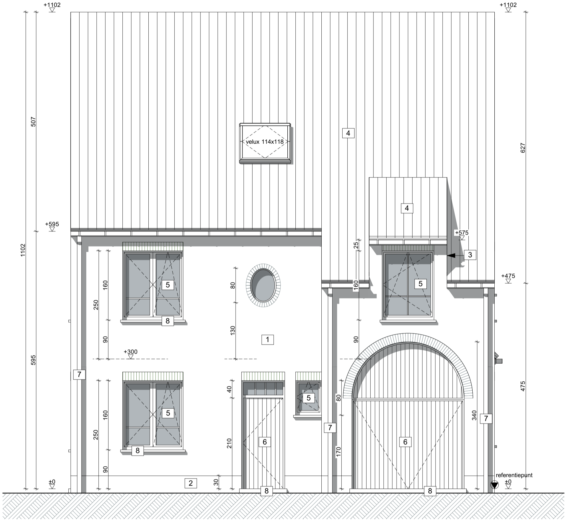
VOORGEVEL
