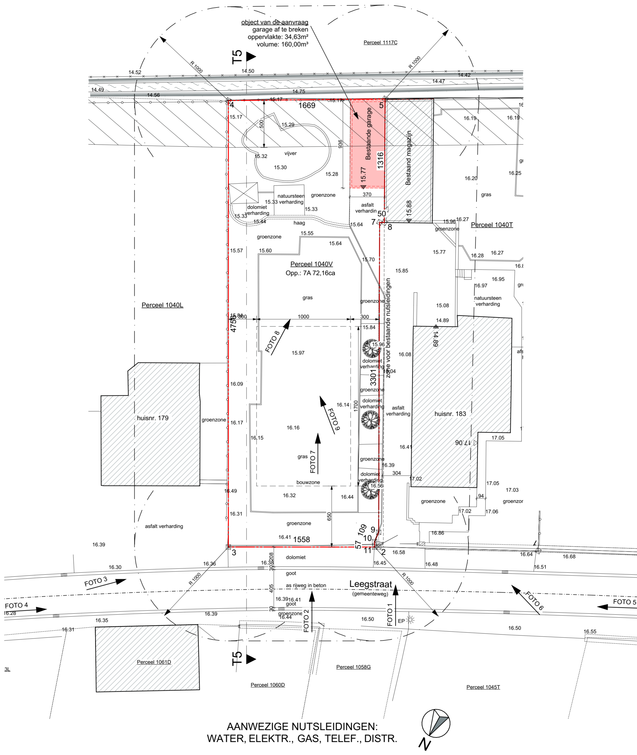
INPLANTINGSPLAN BESTAANDE TOESTAND
