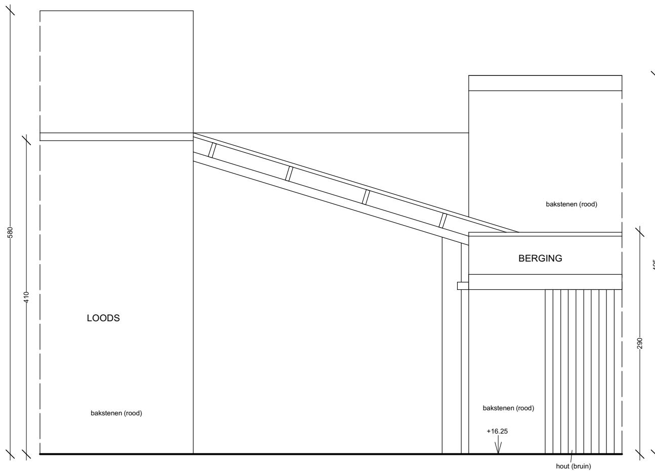
GEVEL noordwest AFDAK schaal 1/50
