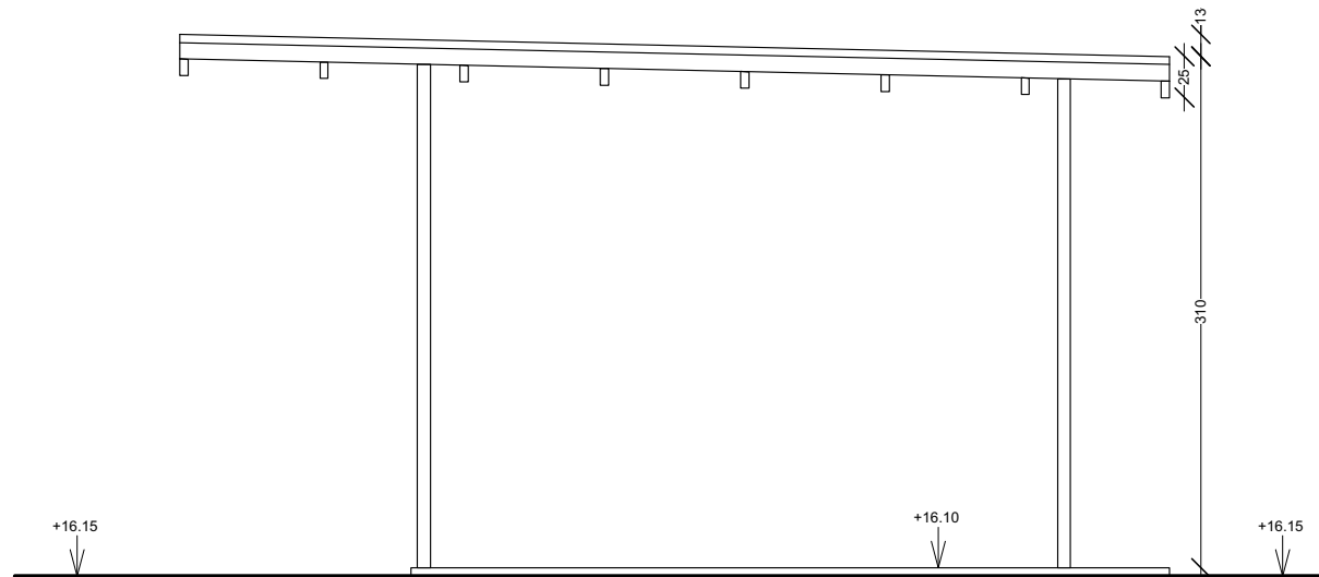
GEVEL noordwest CARPORT schaal 1/50
