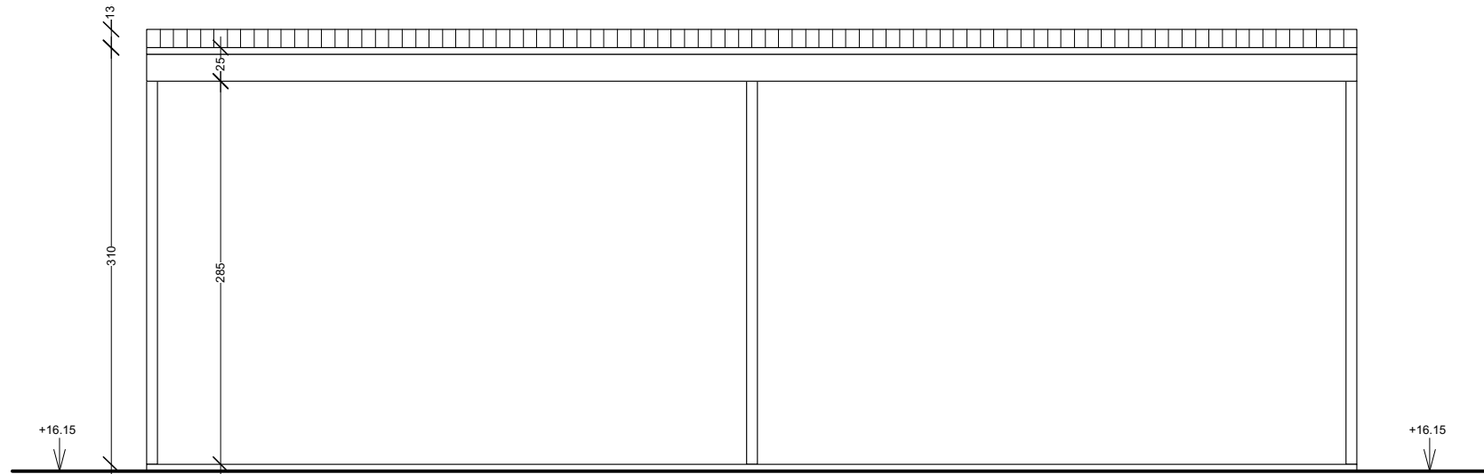
GEVEL zuidwest CARPORT schaal 1/50
