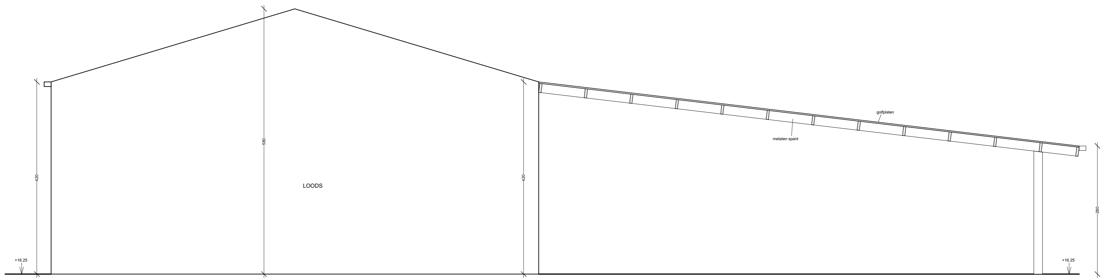
DOORSNEDE CC AFDAK schaal 1/50
