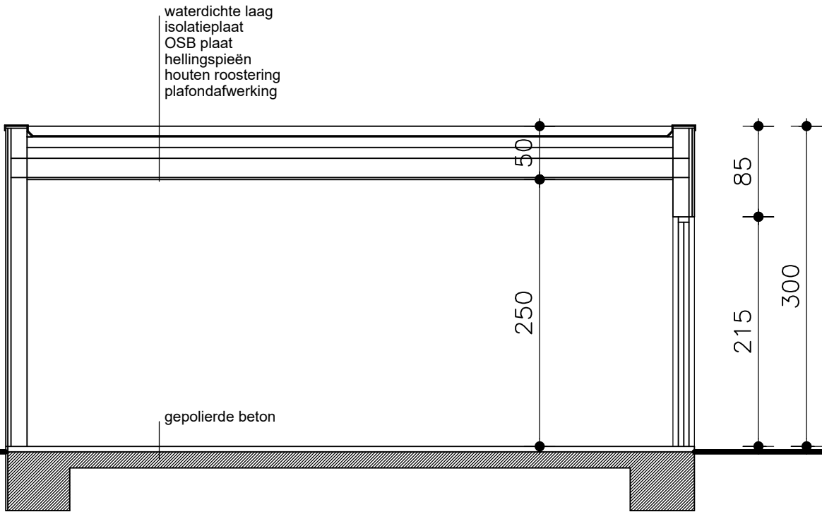
Snede tuinhuis
