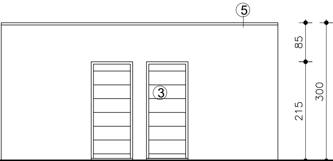
Achtergevel tuinhuis
