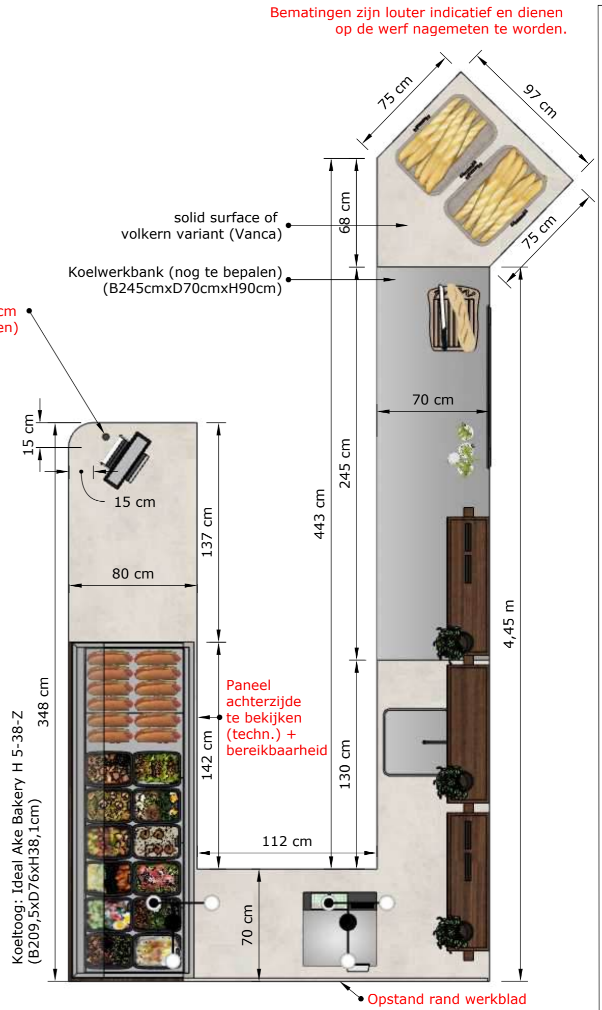
Grondplan
