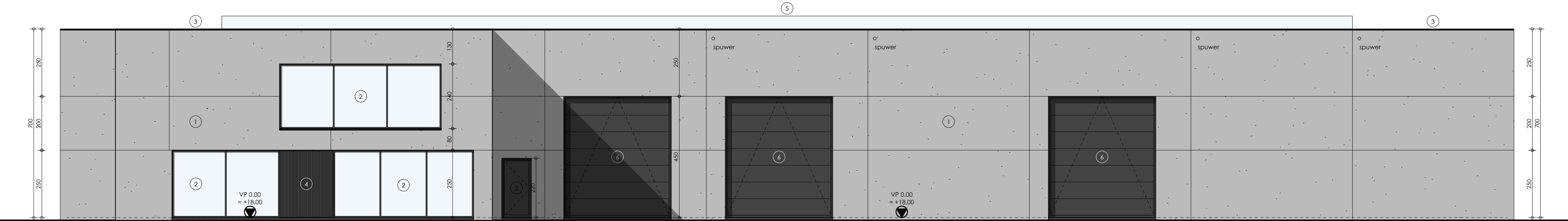
VOORGEVEL schaal 1:100
