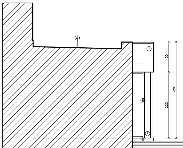
zijaanzicht uitbouw (verspringing) nieuwe uitbouw
