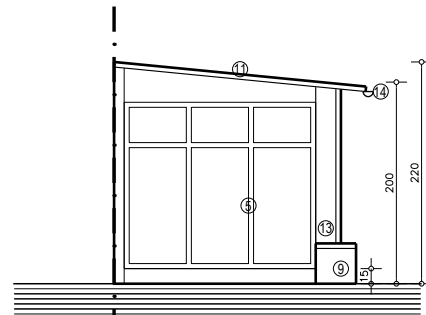
achtergevel nieuwe toestand
