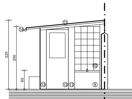
voorgevel nieuwe toestand
