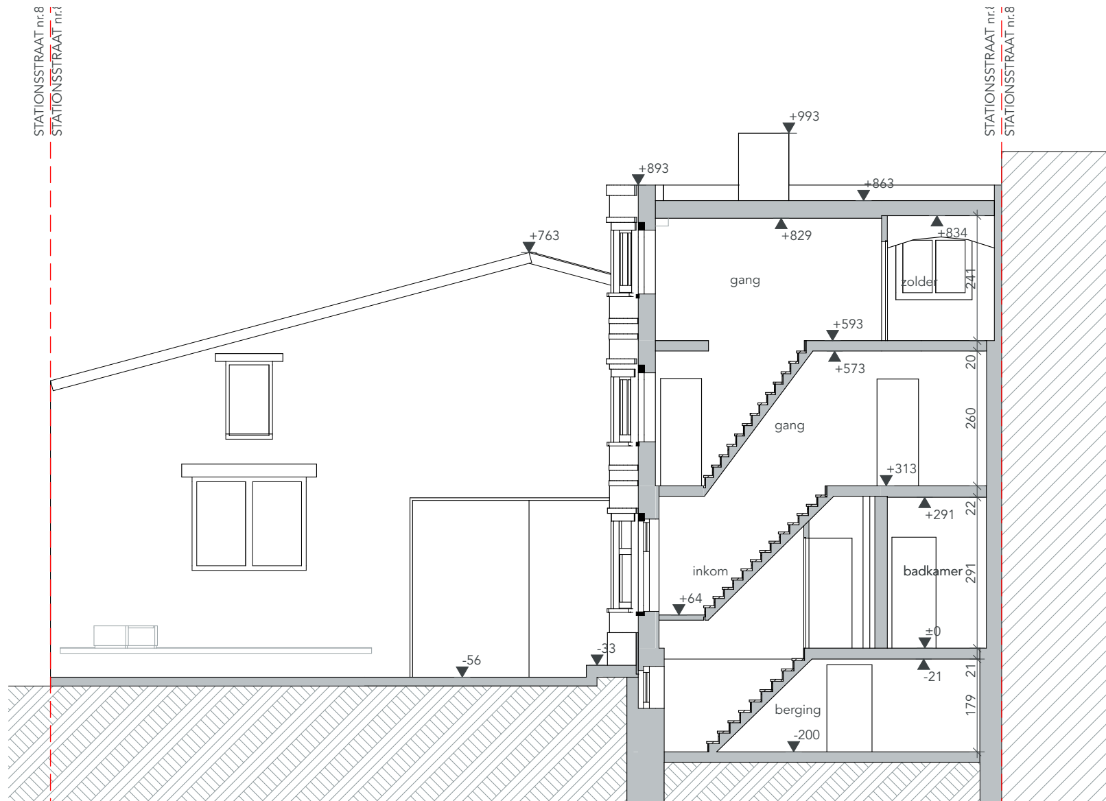
BT Doorsnede A-A
