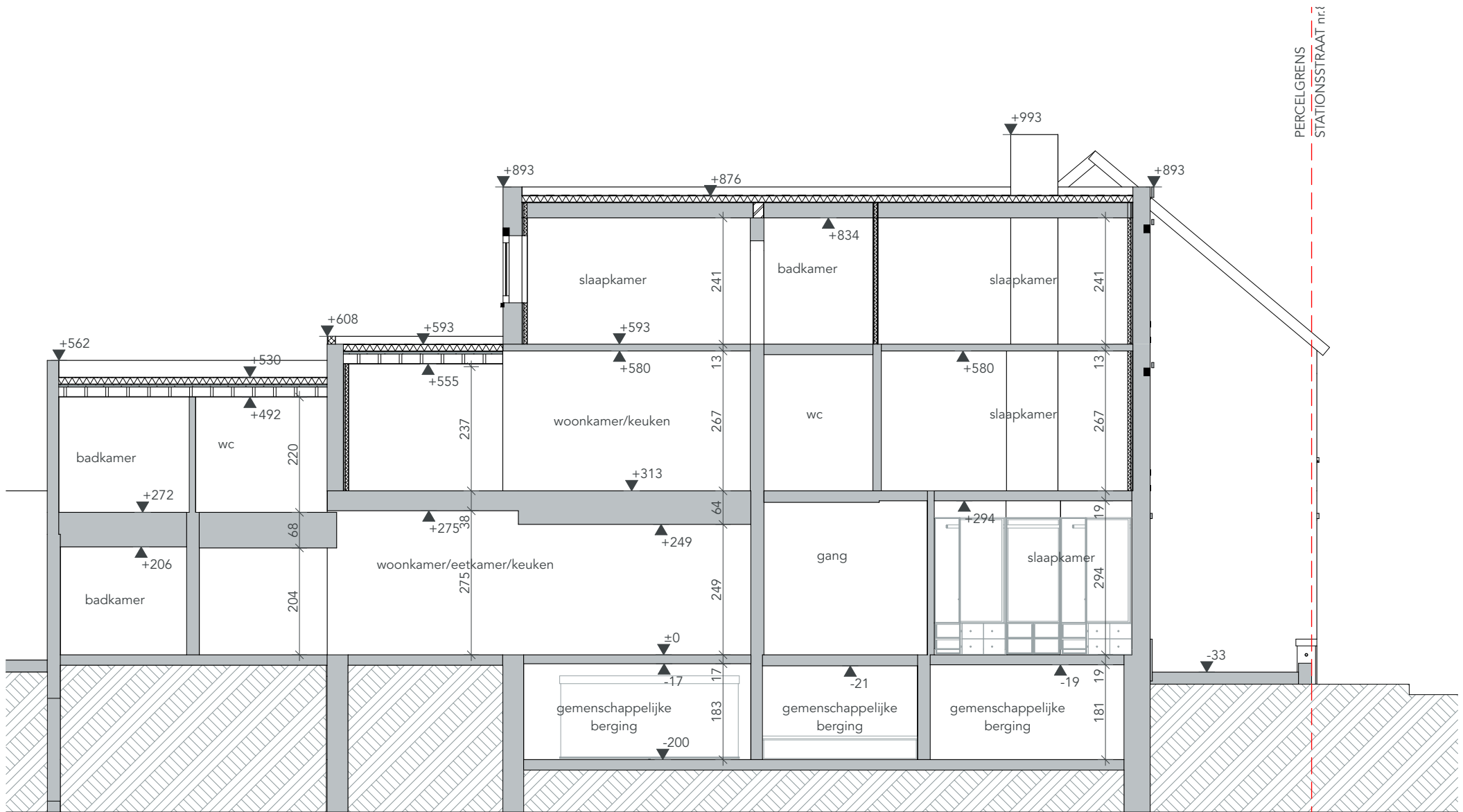
NT Doorsnede B-B
