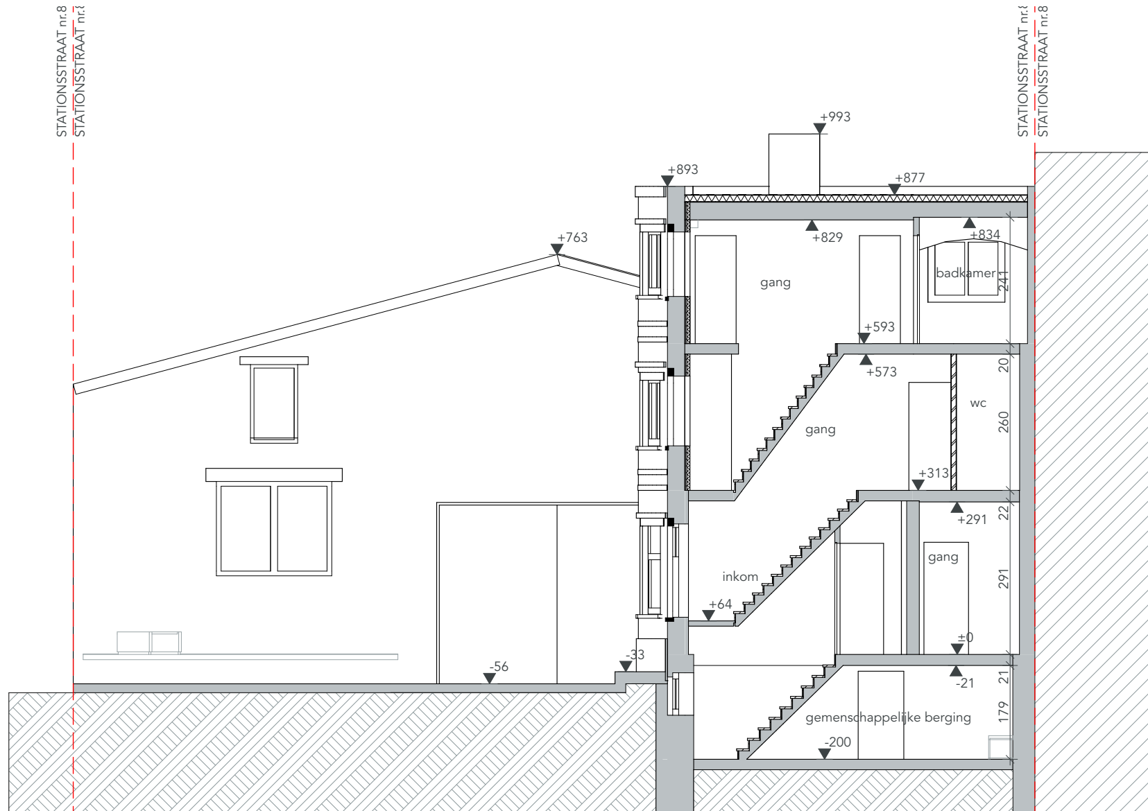
NT Doorsnede A-A
