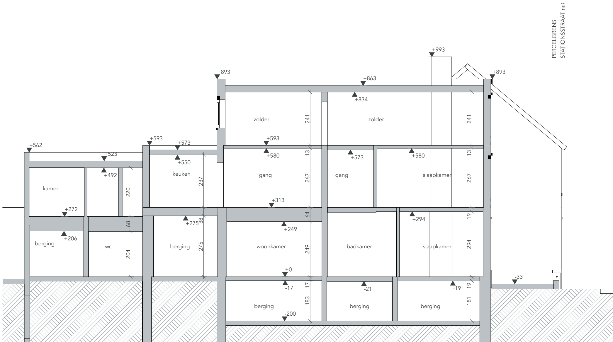
BT Doorsnede B-B
