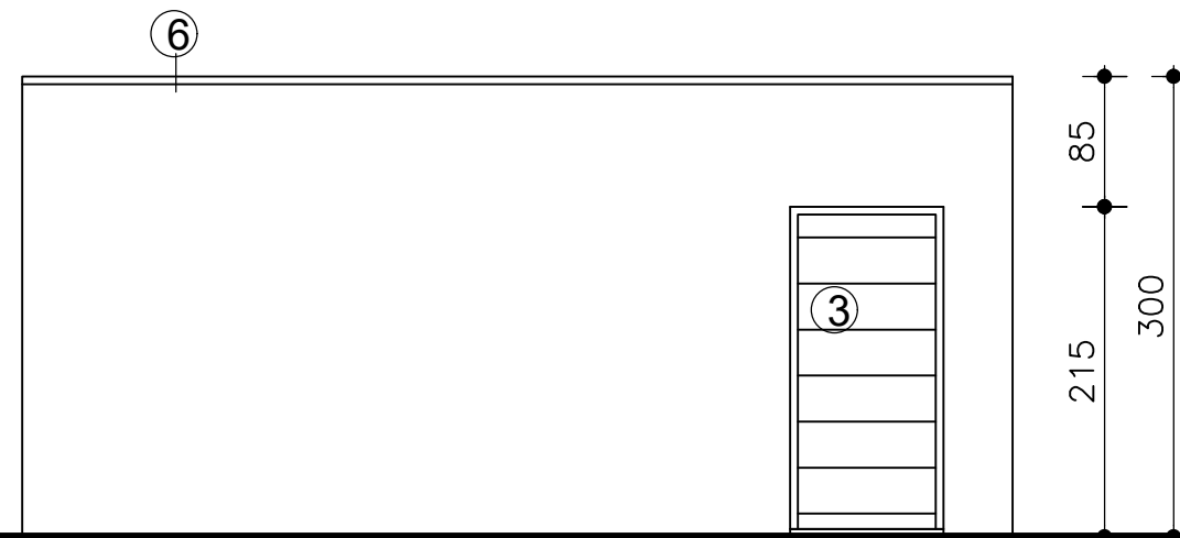
Zijgevel rechts garages 3 en 4
