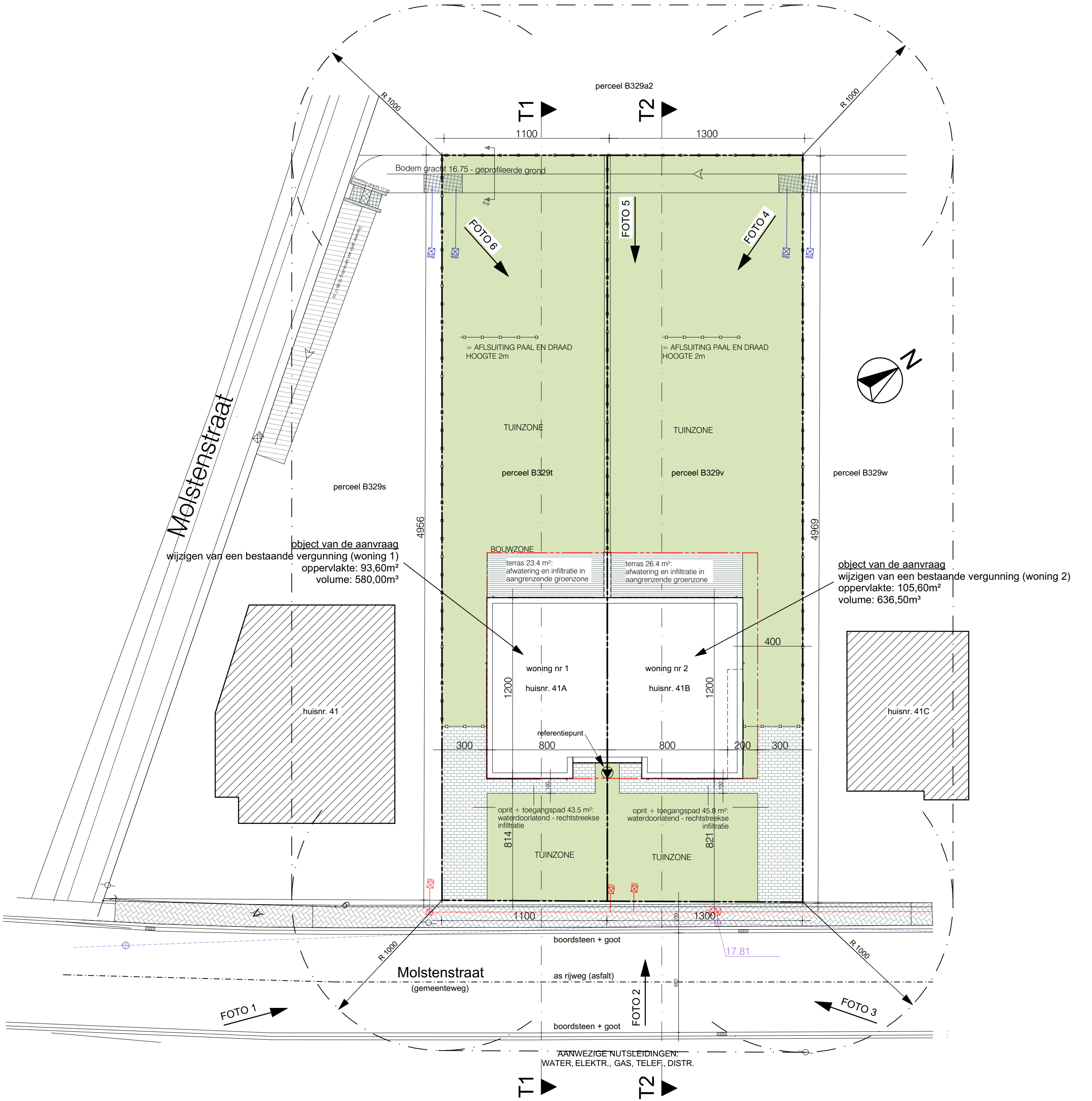
INPLANTINGSPLAN (vergunde toestand) 1:200
