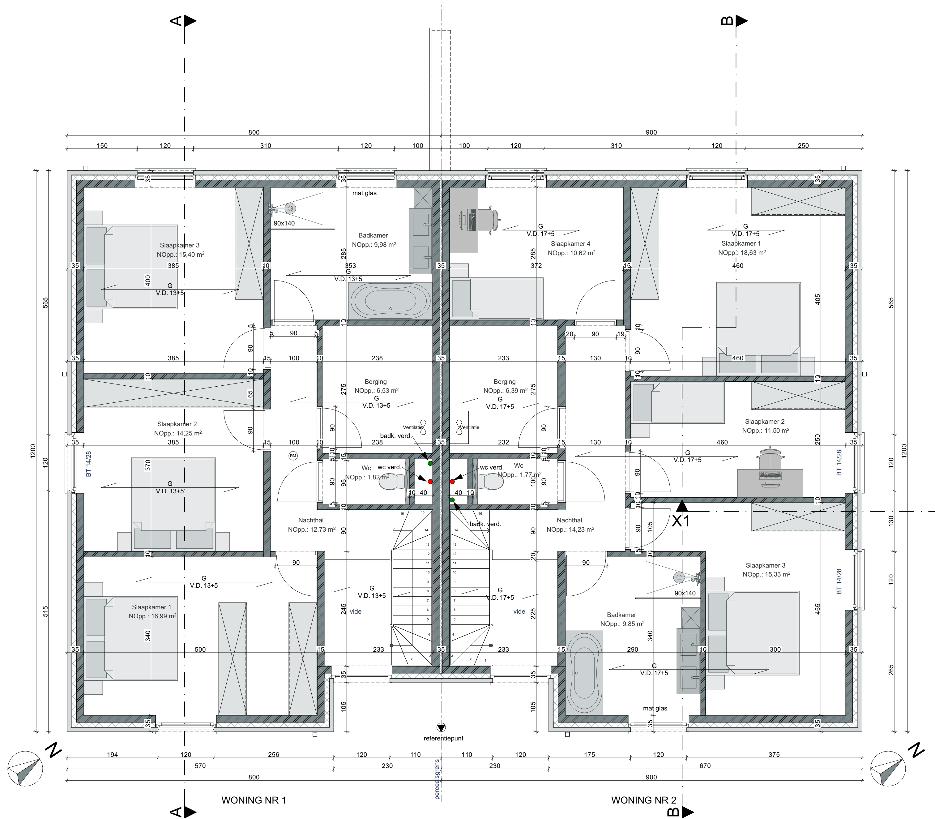
GRONDPLAN VERDIEPING 1 (nieuwe toestand)
