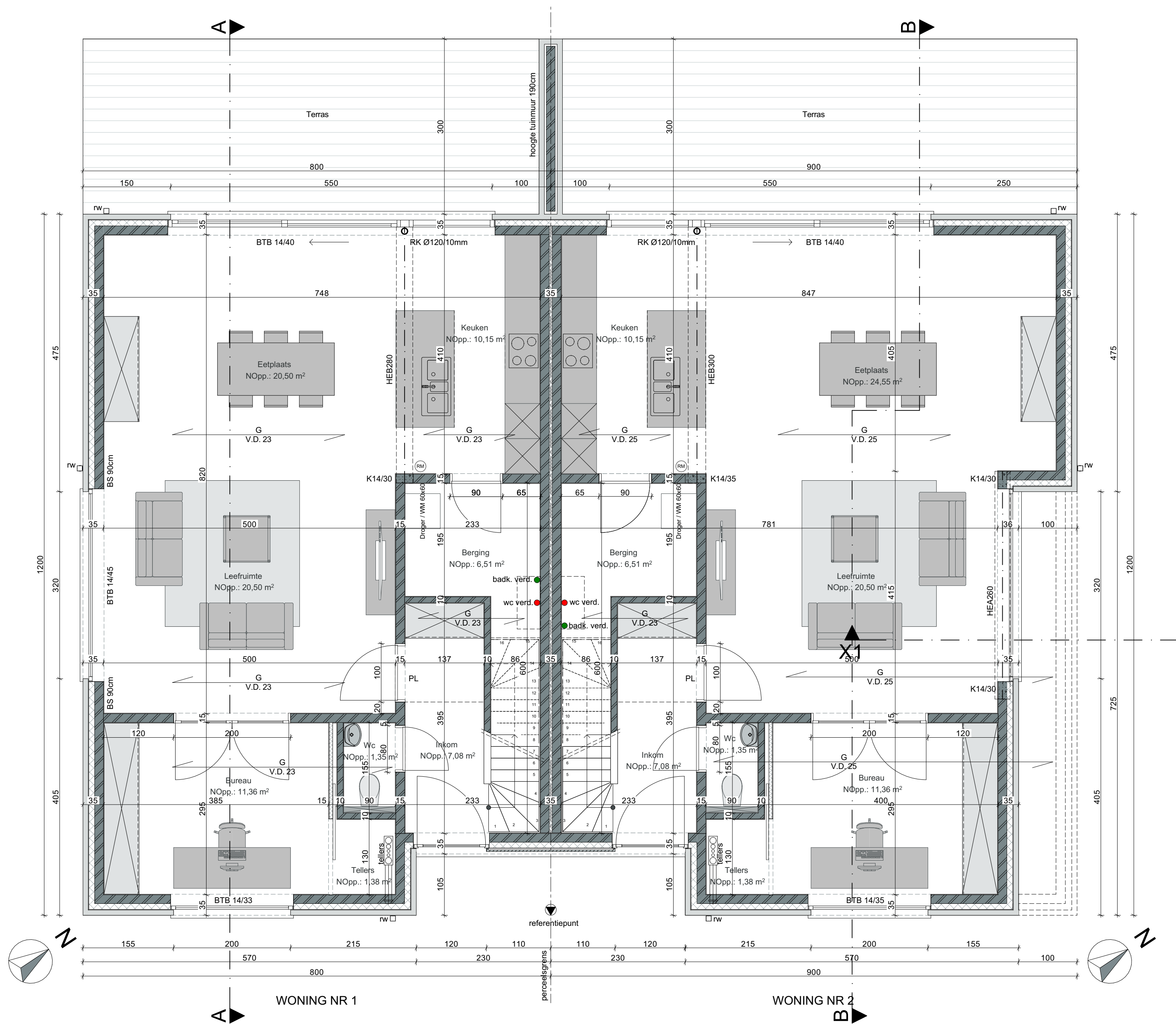
GRONDPLAN GELIJKVLOERS (nieuwe toestand)
