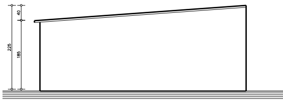
zijgevel rechts gebouw 4 - bestaande toestand
