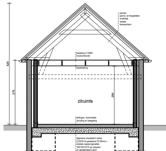
doorsnede ZZ gebouw 3 - nieuwe toestand
