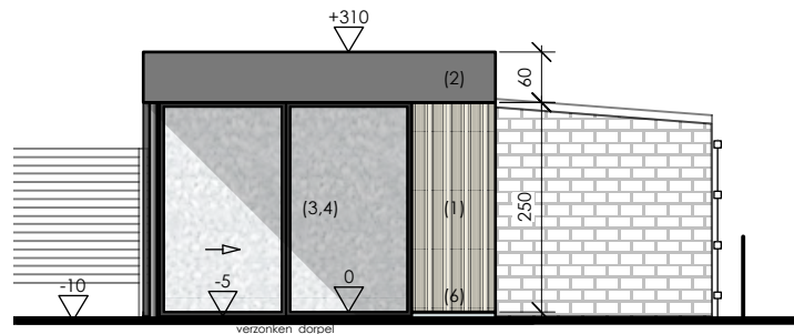
RECHTERGEVEL (ZUID)
