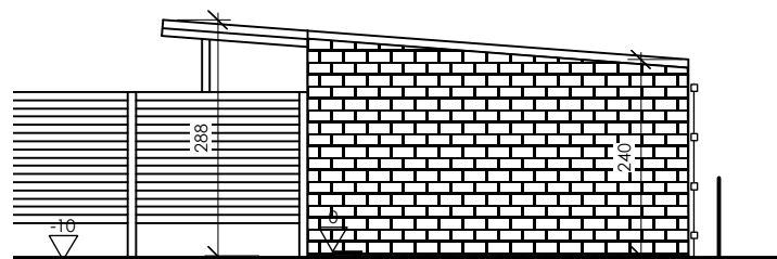
GABARIT nr 130
