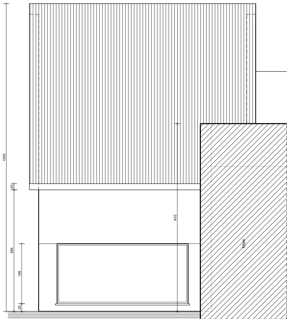
zijgevel rechts bestaande toestand
