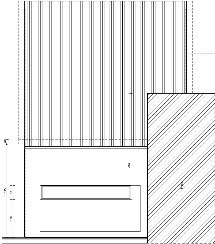
zijgevel rechts nieuwe toestand
