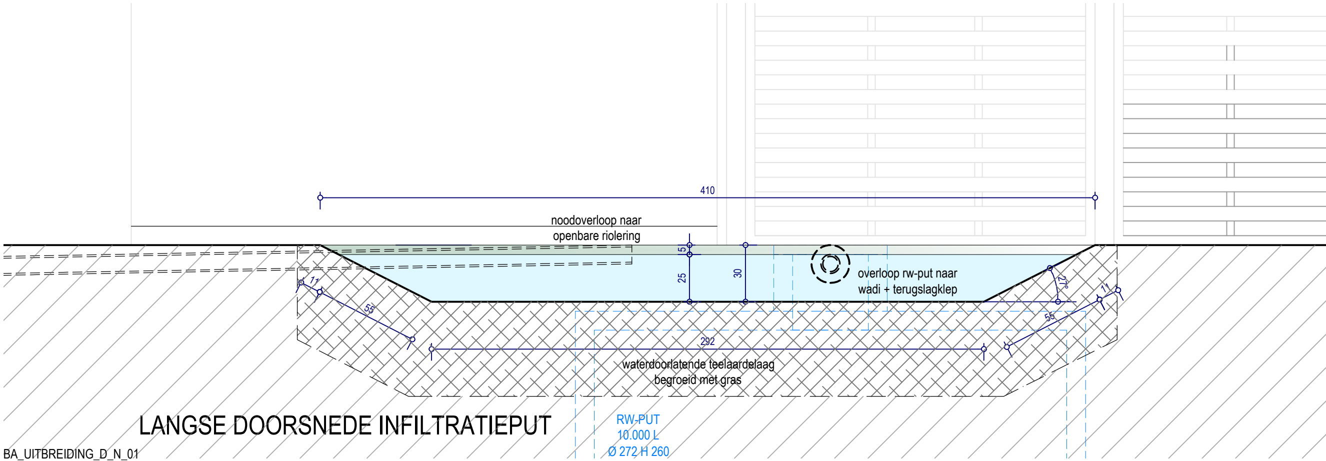
DWARSE DOORSNEDE INFILTRATIEPUT
