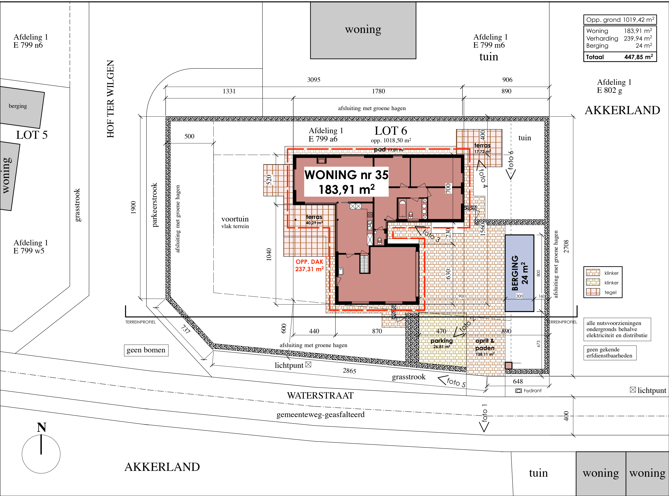
INPLANTINGSPLAN BESTAAND 1/200
