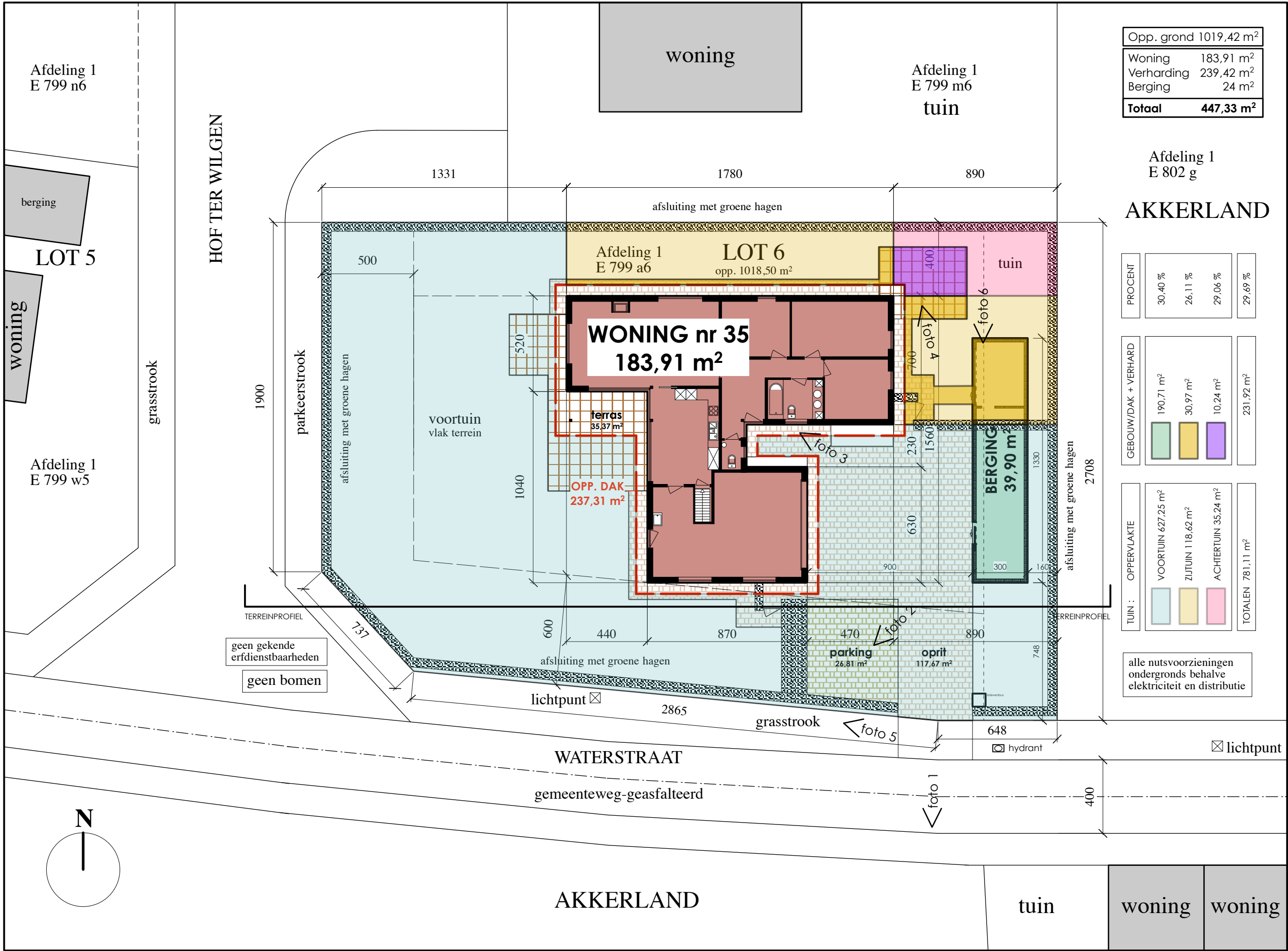
PLAN TUINZONES NIEUW (met oversteek) 1/200
