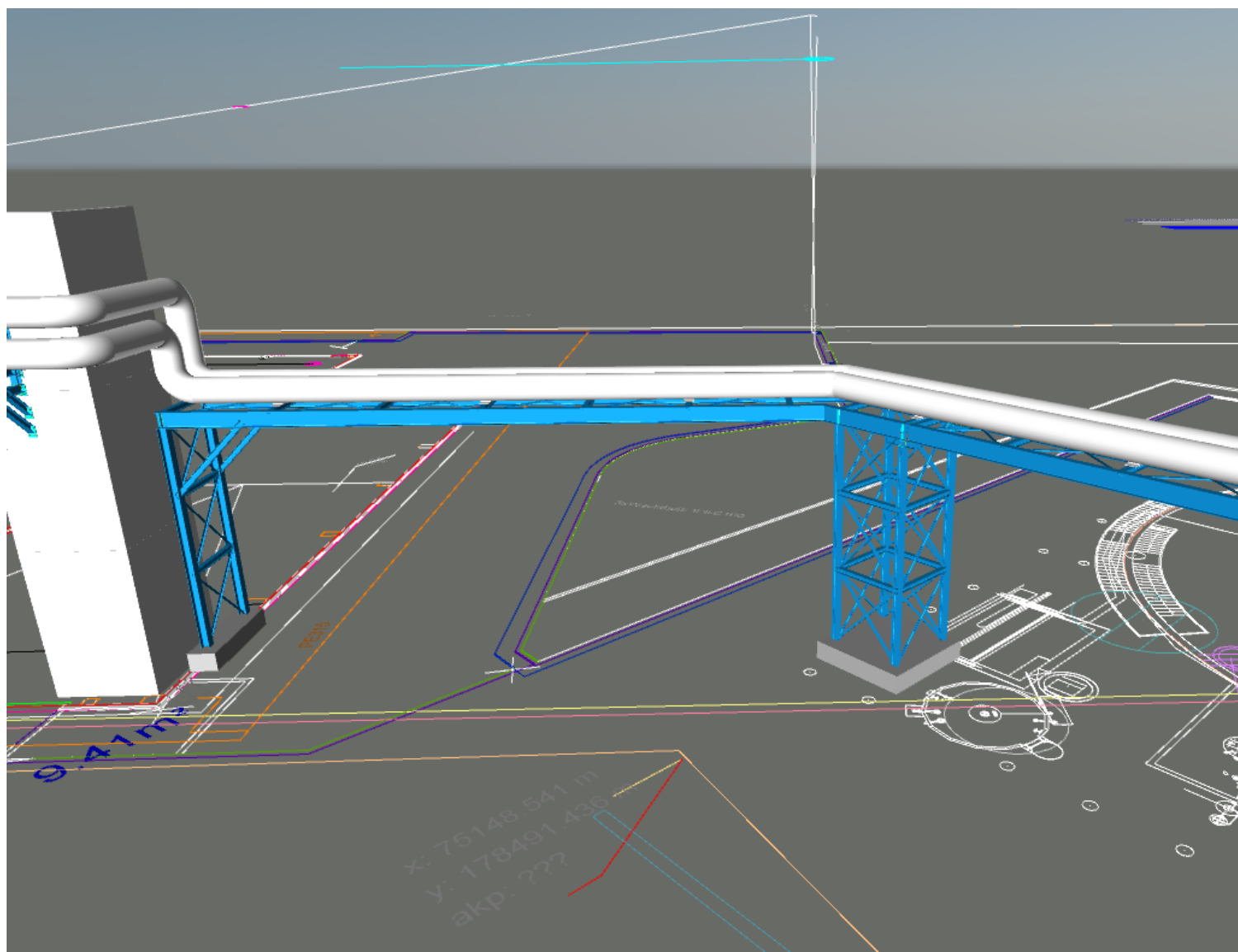
Piperack 3 langs portiersgebouw en waterzuivering naar hal 12 (detail) (3) – peil hoogte leidingen : + 8,95m
