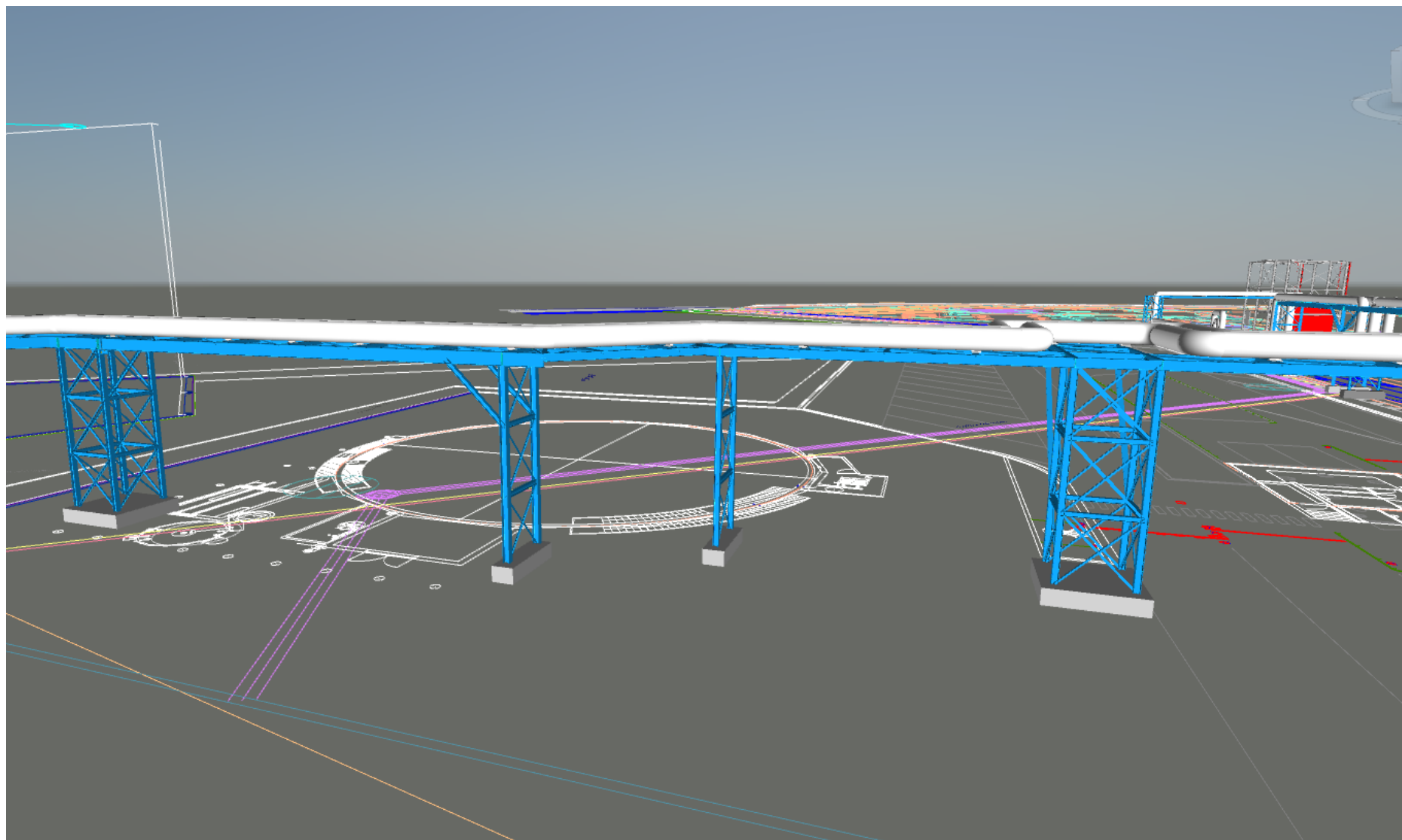
Piperack 3 langs portiersgebouw en waterzuivering naar hal 12 (detail) (2) – peil hoogte leidingen : + 8,95m
