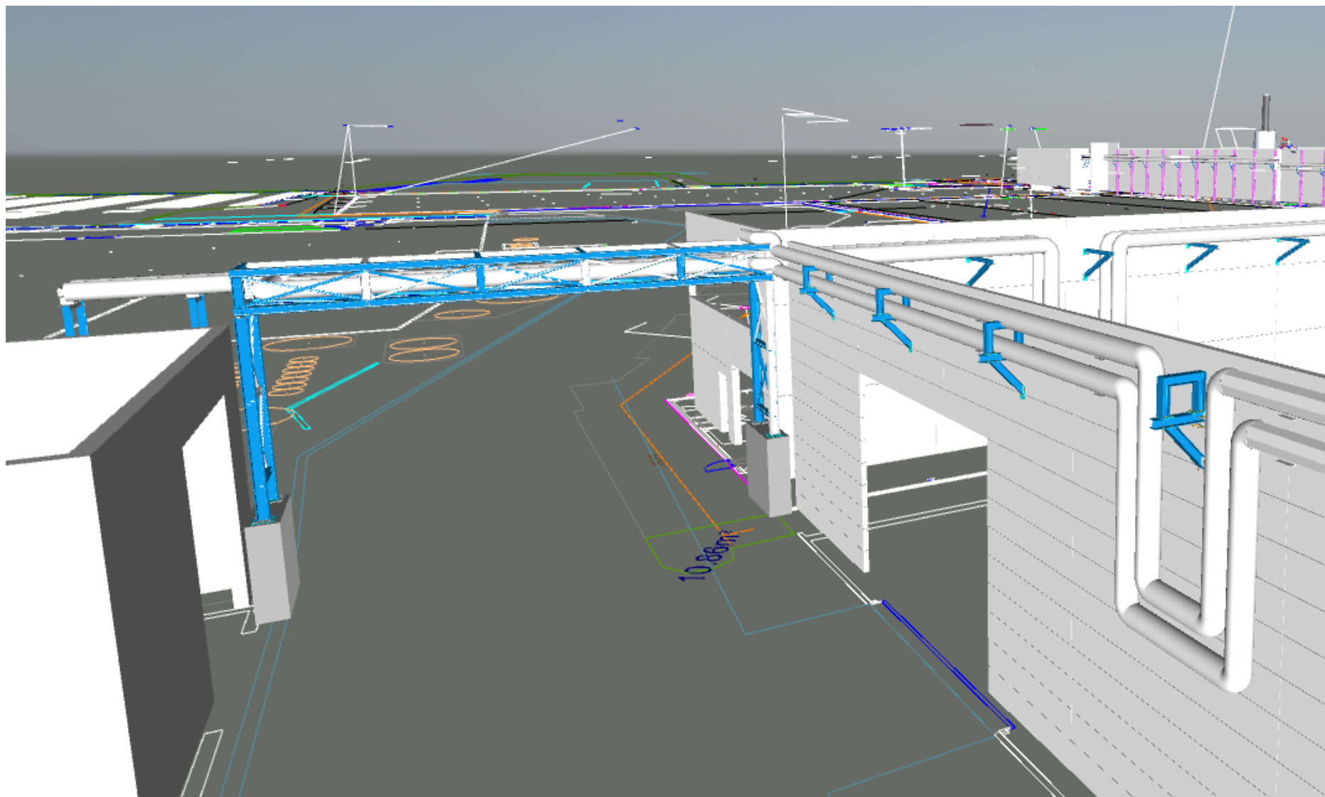
Piperack gebouw labo/engineering – aftakking naar tie-ins pers 4
