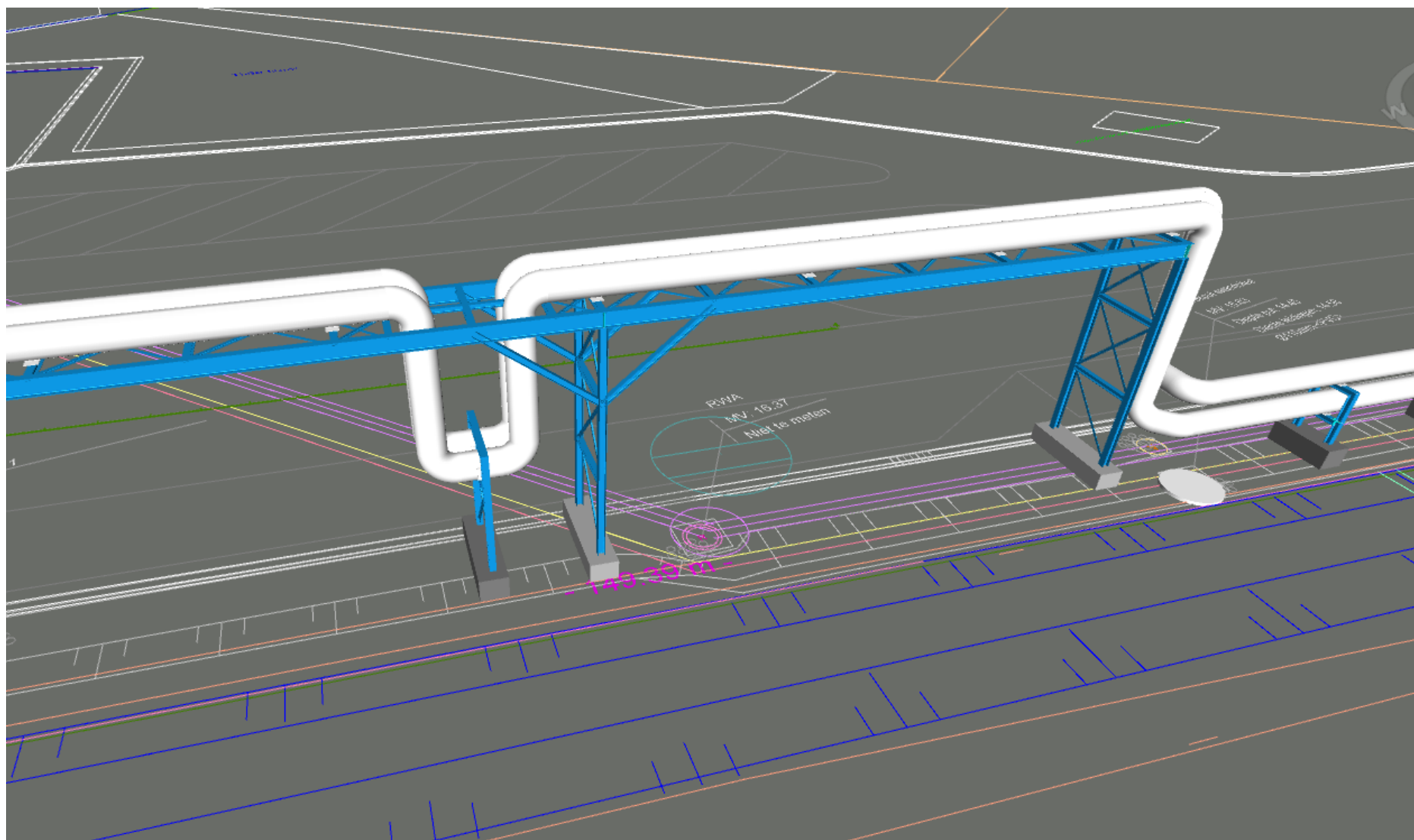
Detail piperack 3 peil bovenzijde leidingen : +8,95m
