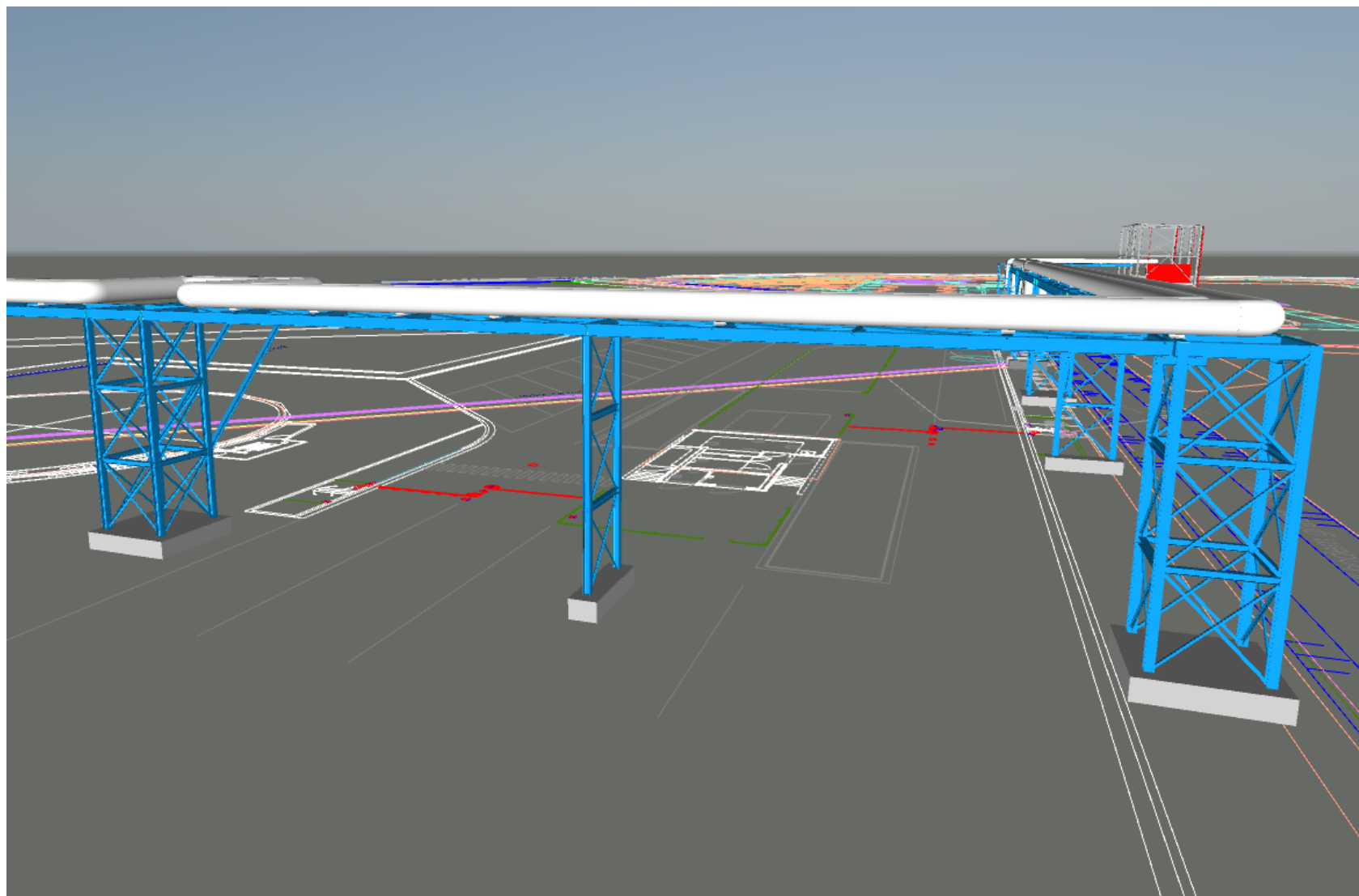
Piperack 3 langs portiersgebouw en waterzuivering naar hal 12 (detail) (1) – peil hoogte leidingen : + 8,95m
