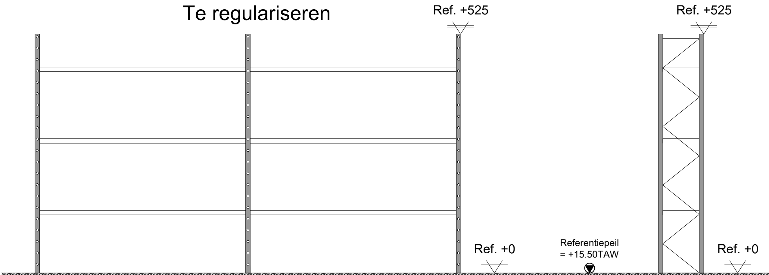
PRINCIPETEKENING Onoverdekte rekken 2 -1/50-
