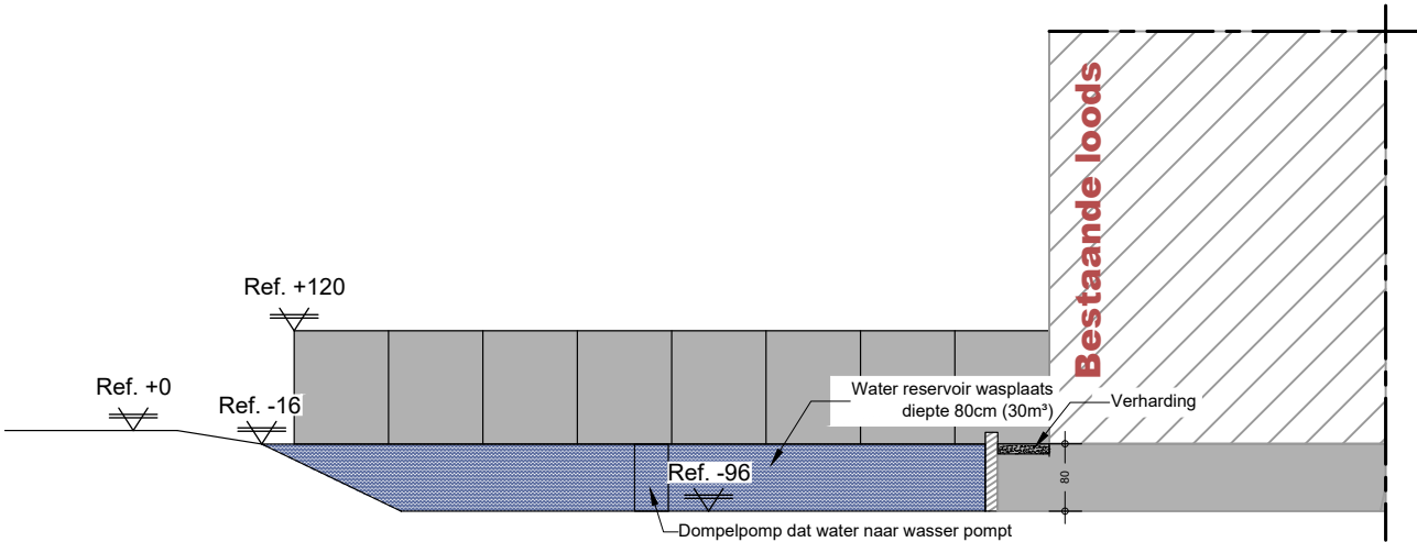
PRINCIPETEKENING WASPLAATS LAVA -1/100-
