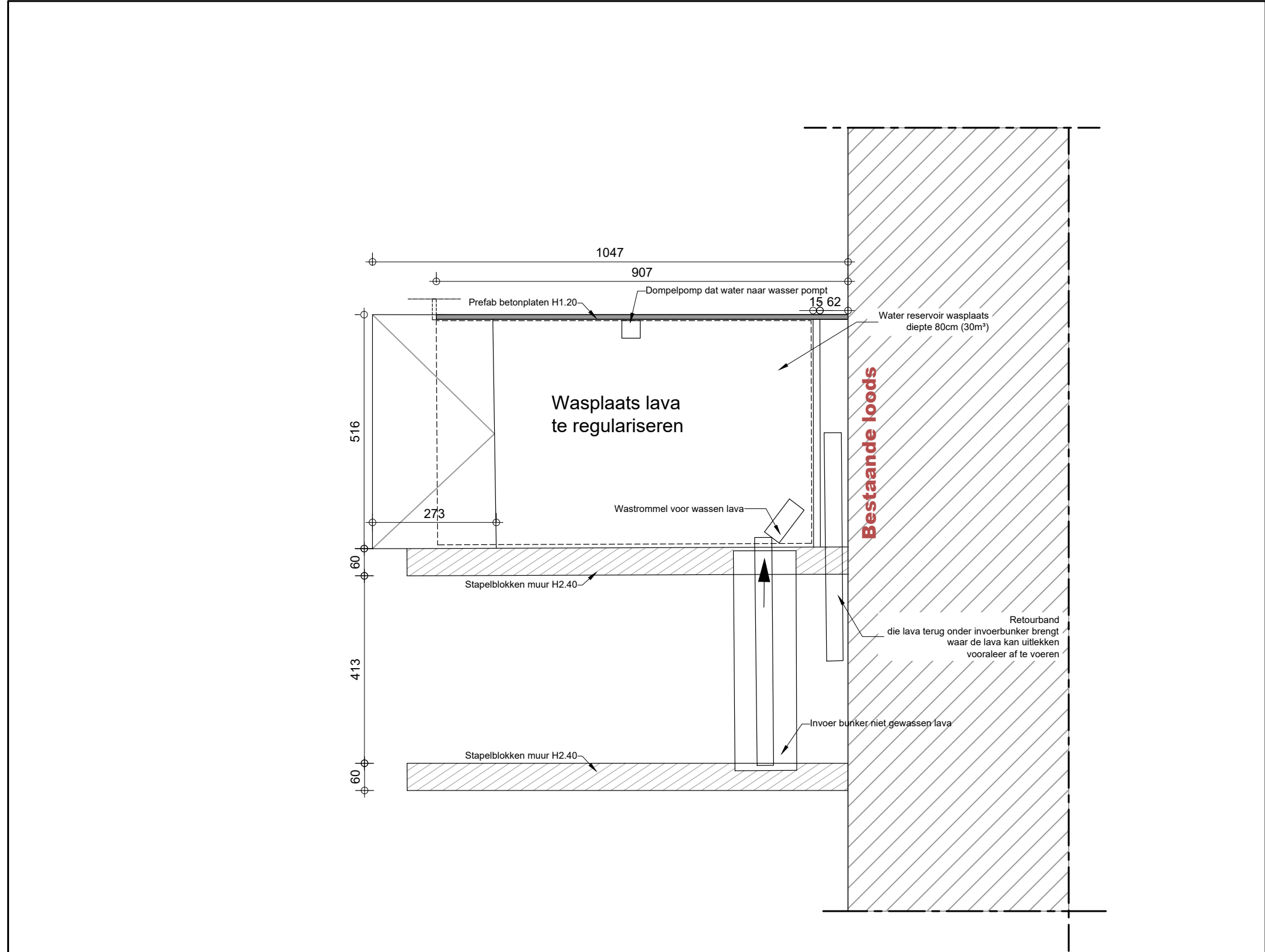
GRONDPLAN WASPLAATS LAVA -1/100-
