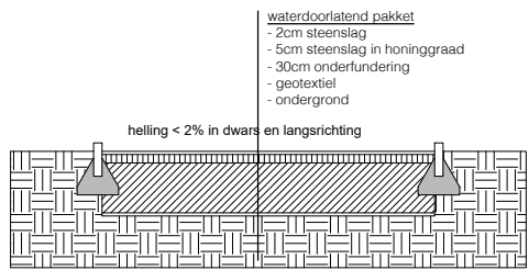
opbouw waterdoorlatende verharding
