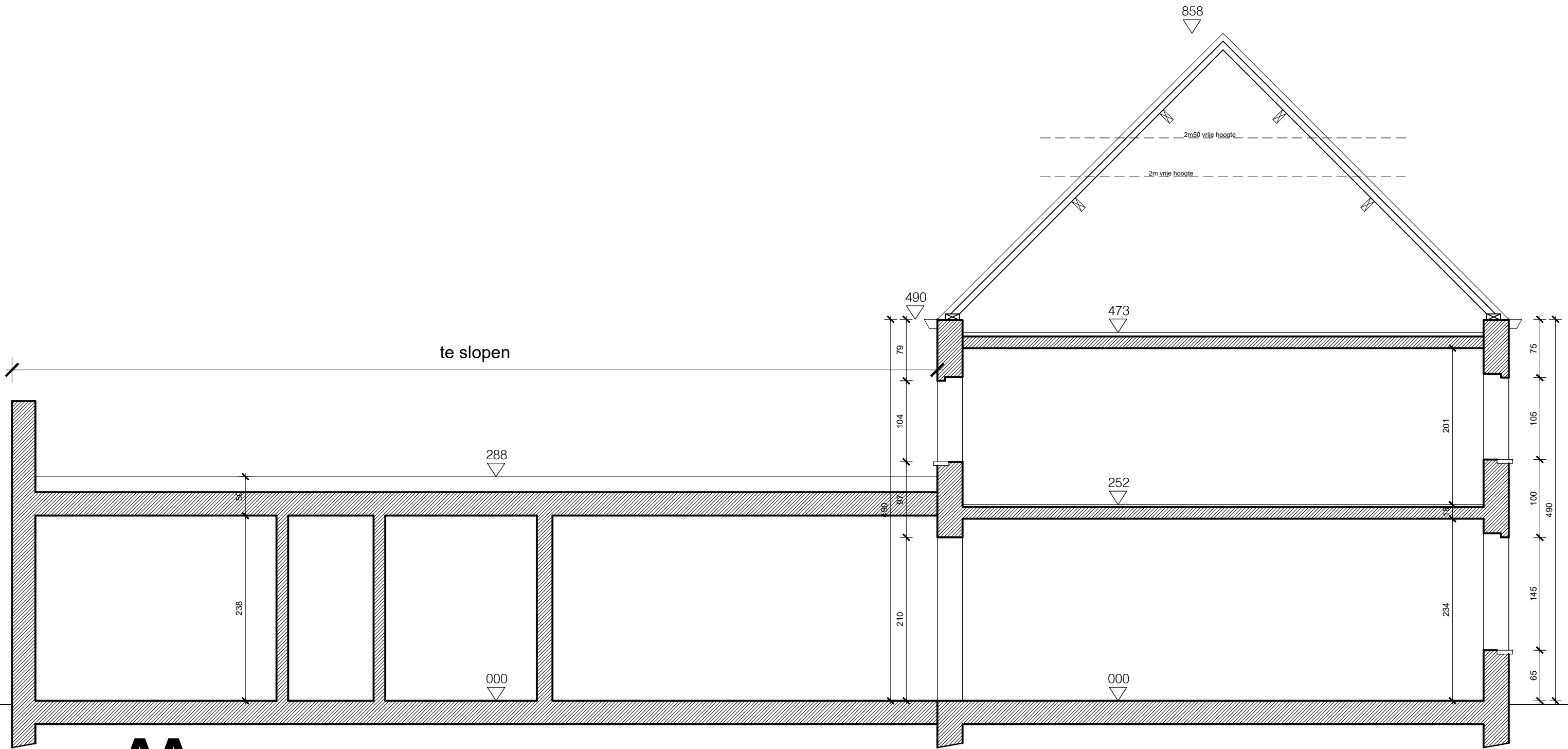
snede AA 1/50 bestaande toestand
