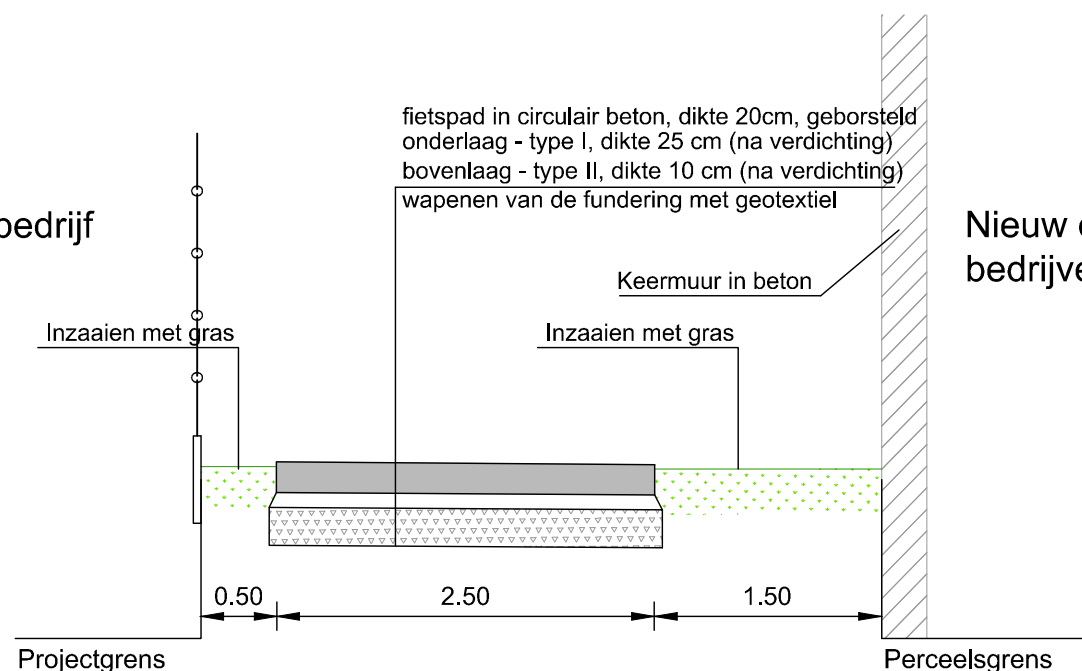
Type dwarsprofiel fietspad
