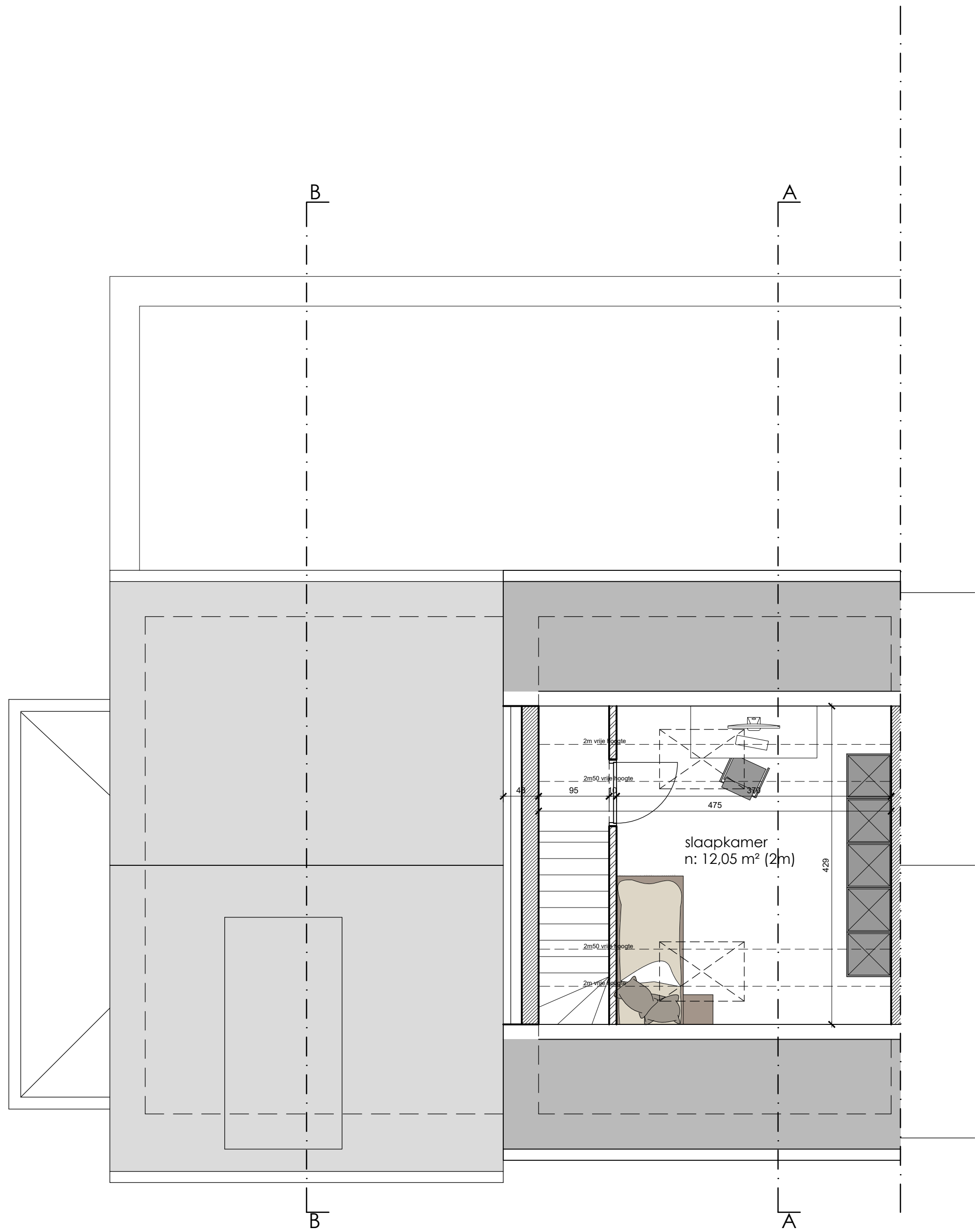
plan VERDIEPING +2 1/50 nieuwe toestand
