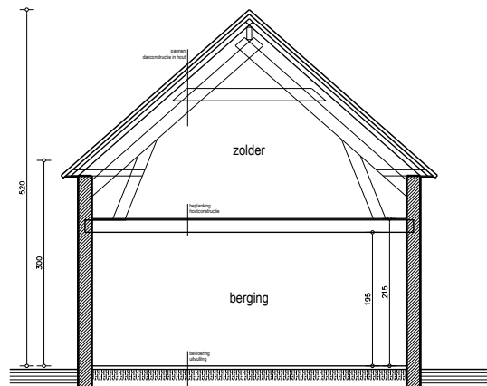
doorsnede gebouw 3 - bestaande toestand
