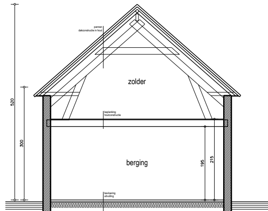
doorsnede gebouw 3 - nieuwe toestand
